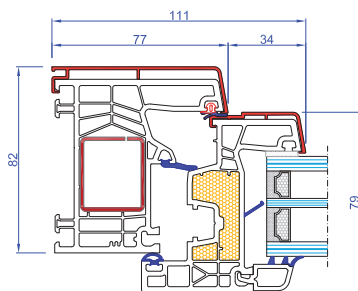
Telaio a "L"
