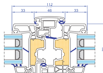
Nodo centrale asimmetrico
