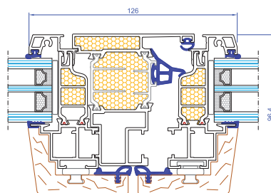
Nodo centrale Simmetrico
