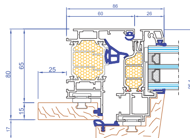
Telaio con aletta da 25mm
