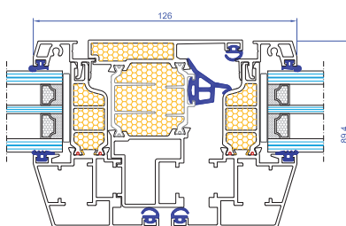
Nodo centrale Simmetrico
