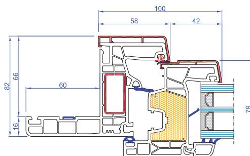
Telaio da ristrutturazione con aletta da 60mm
