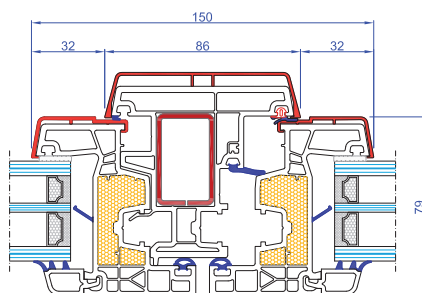
Nodo centrale simmetrico
