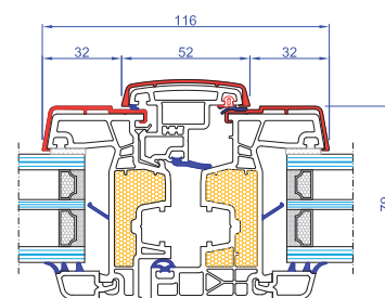
Nodo centrale asimmetrico
