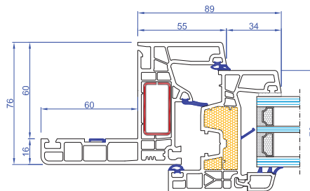
Telaio da ristrutturazione con aletta da 60mm
