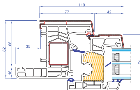
Telaio con aletta da 35mm
